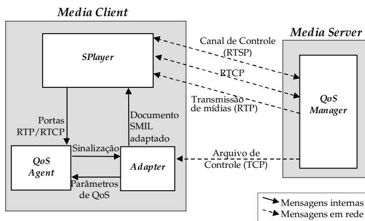
Figura 11 – Módulos principais da arquitetura do Projeto ServiMídia. [16]
