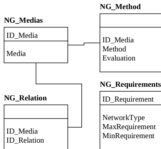
Figura 16 – Modelagem do Banco de Parâmetros
