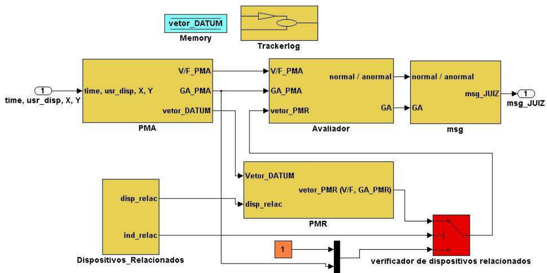
Figura 4.5. Diagrama em blocos Simulink do módulo ANAMOB.
