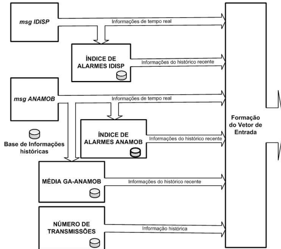
Figura 3.10. Mecanismo de Pré-Processamento de entradas.
