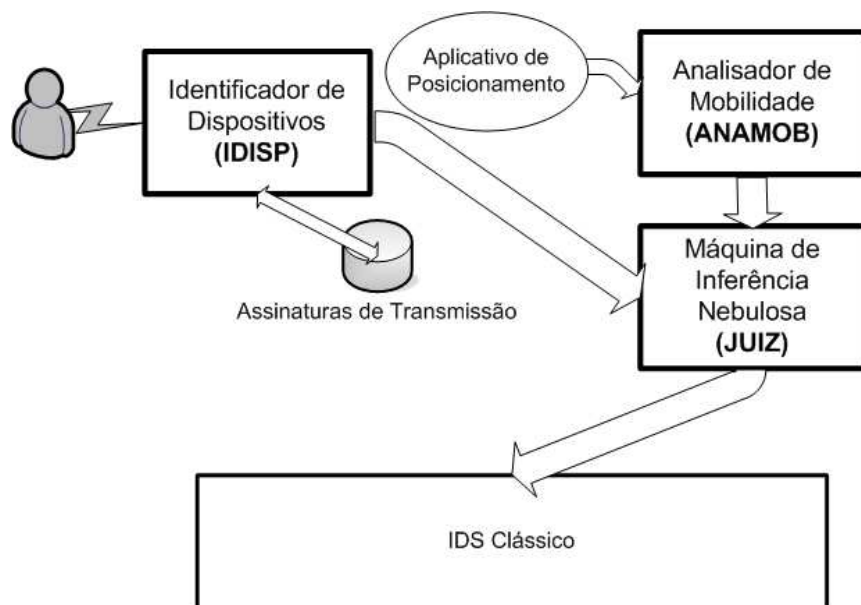
Figura 3.1. Arquitetura EWIDS proposta [13].
