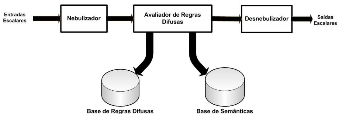
Figura 2.9. Diagrama de um sistema nebuloso.
