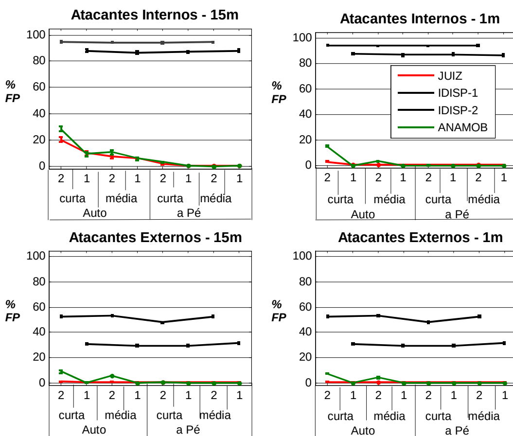
Figura 5.6. Resultados obtidos para Falsos Positivos (FP).
