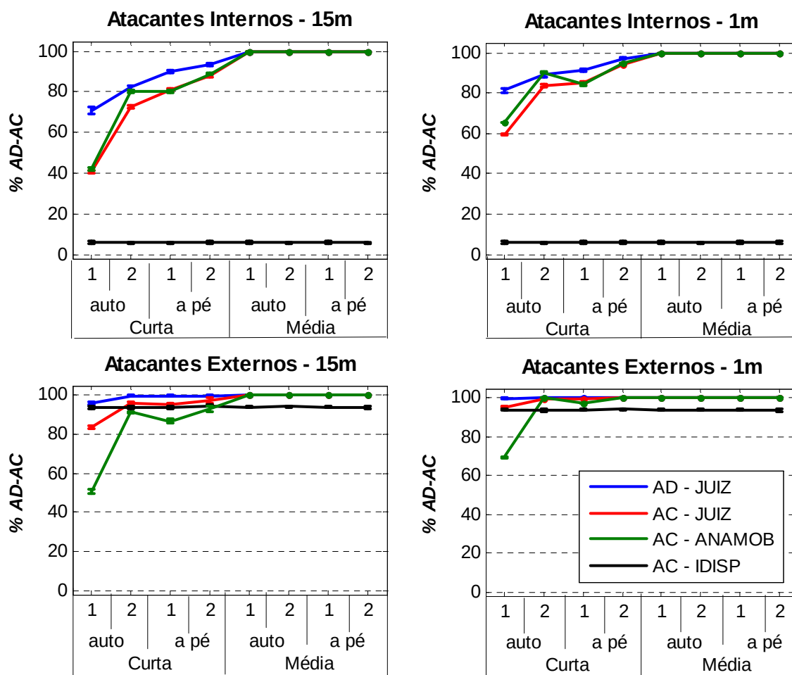
Figura 5.4. Resultados obtidos para Atacantes Descobertos (AD) e Alarmes Corretos (AC).
