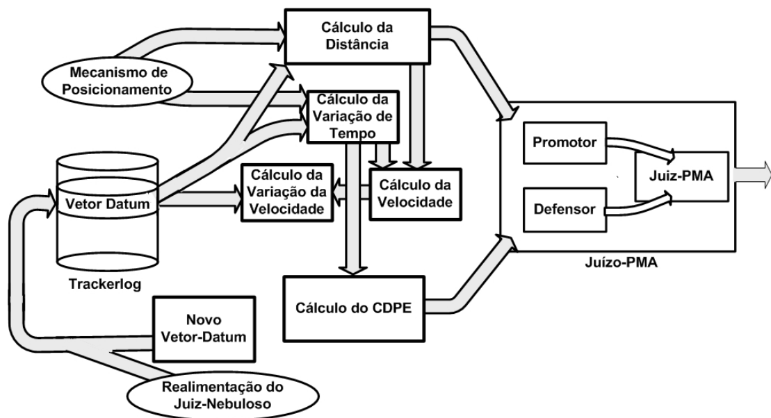
Figura 3.6. Diagrama geral do bloco PMA.
