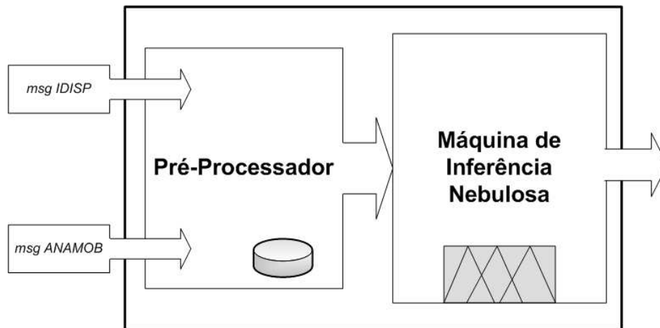
Figura 3.8. Diagrama em blocos do componente JUIZ.
