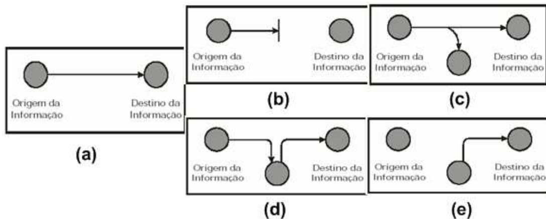
Figura 2.3. (a) Fluxo normal. (b) Fluxo Interrompido. (c) Fluxo interceptado. (d) Fluxo modificado. (e) Fluxo fabricado.
