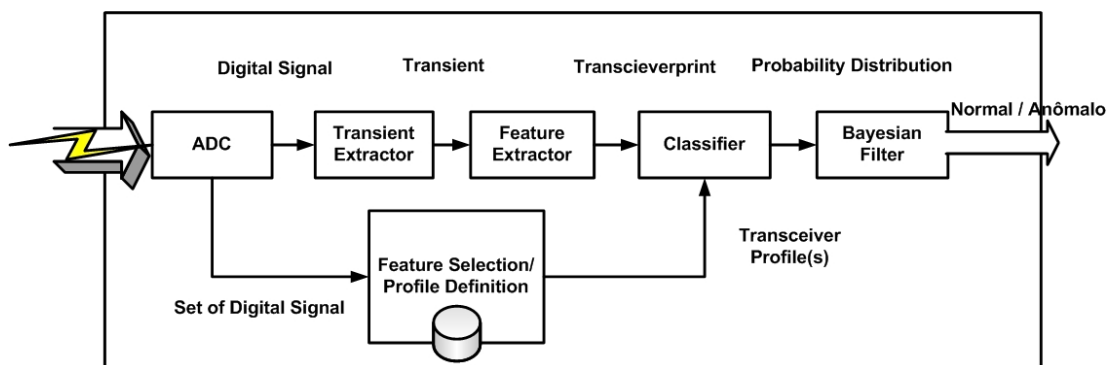
Figura 2.10. Digrama em blocos do componente IDISP.
