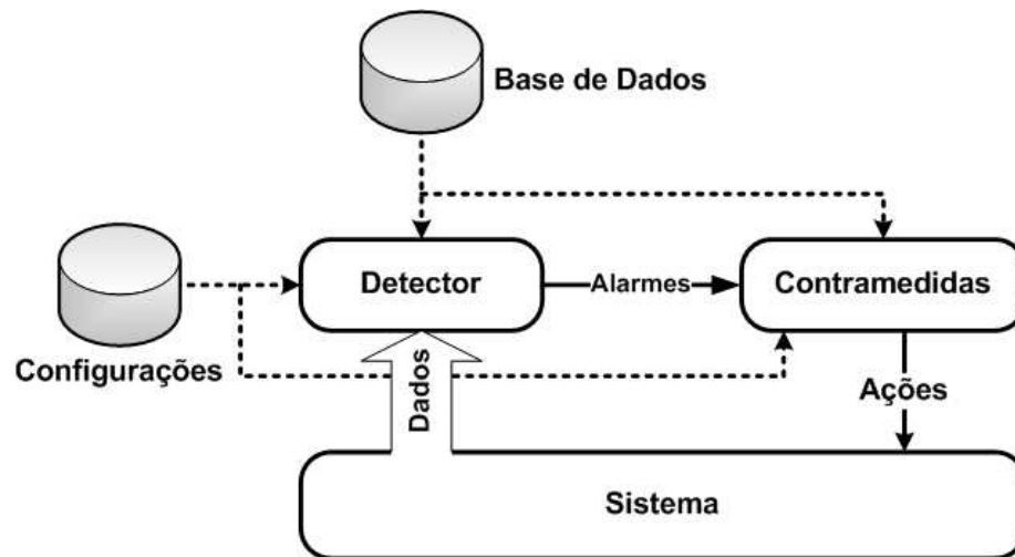
Figura 2.6. Generalização de um IDS [28].
