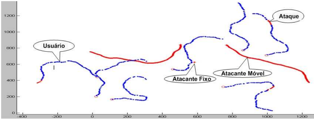
Figura 5.1 - Cenário ilustrativo gerado com sete usuários e três atacantes.
