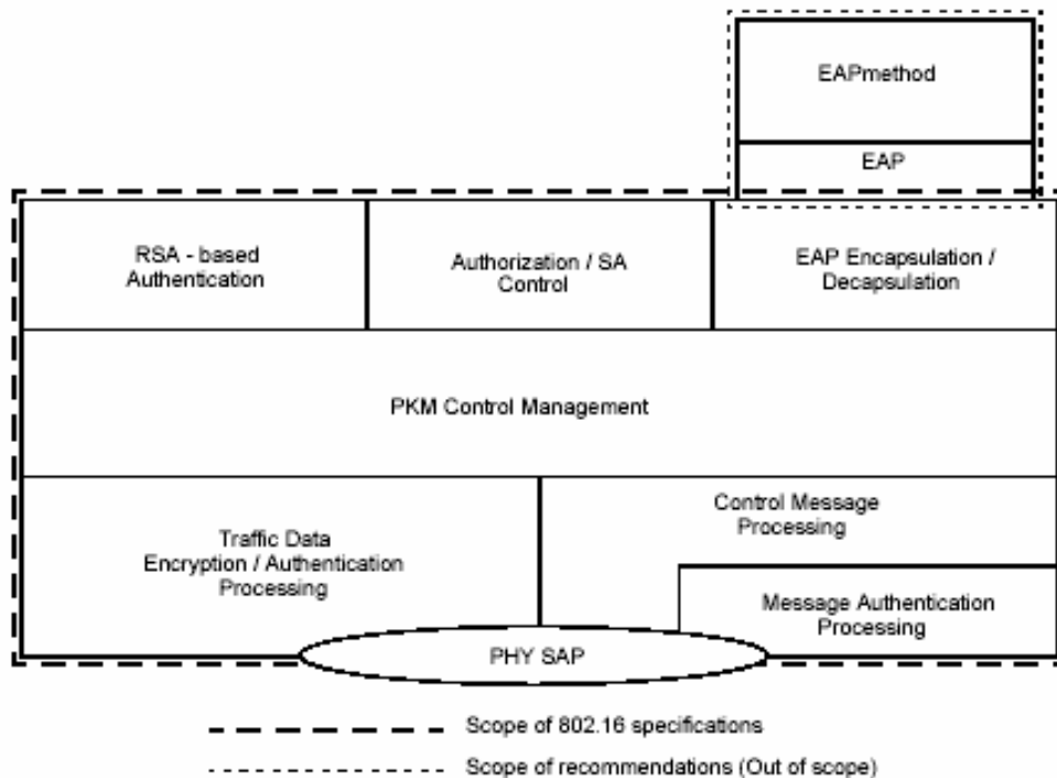
Figura 2.5. Nova Subcamada de Segurança do Padrão IEEE 802.16e [1]
