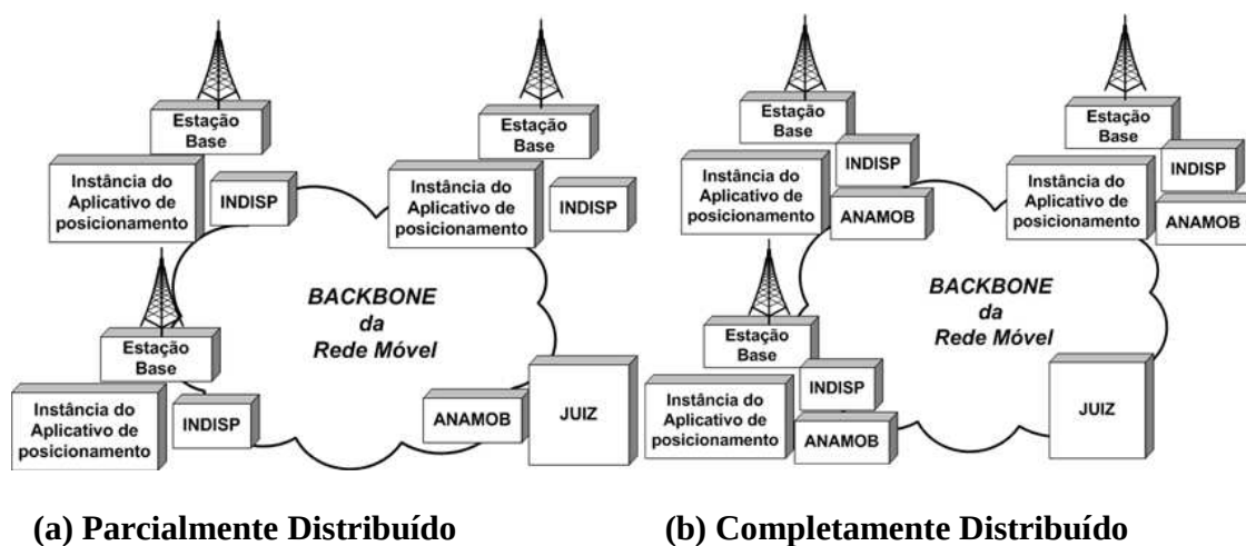
Figura 3.11. Organização dos componentes da Arquitetura EWIDS.
