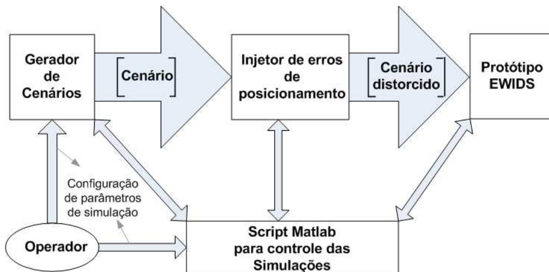
Figura 4.1. Esquema geral de controle das simulações.
