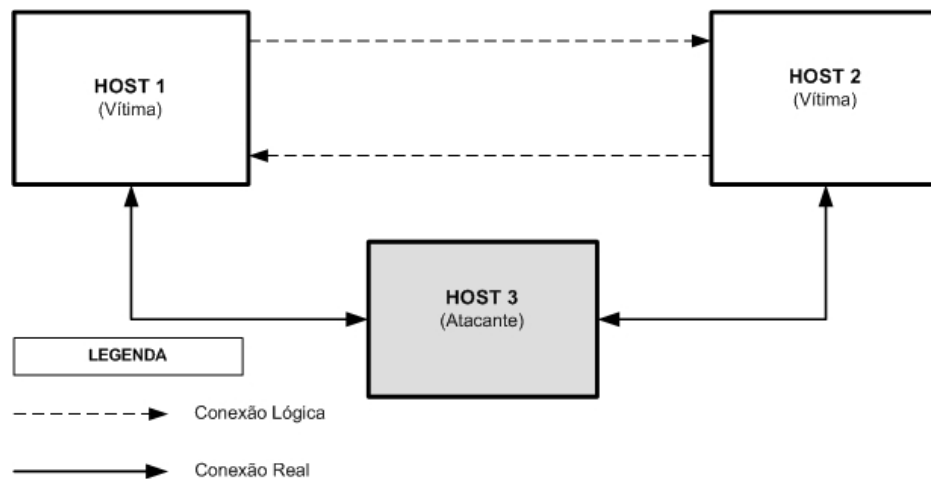
Figura 2.4. Ataque de man-in-the-middle.
