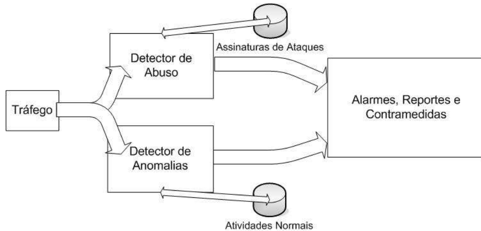
Figura 2.7. Métodos de Detecção contidos em uma Arquitetura clássica de IDS.
