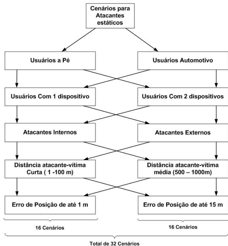
Figura 5.2 – Diagrama de formação de Cenários de Simulação.
