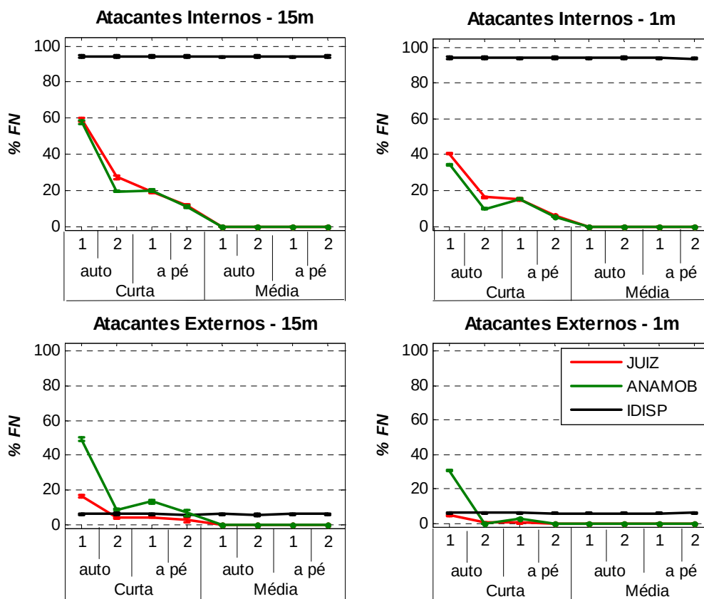
Figura 5.5. Resultados obtidos para Falsos Negativos (FN).
