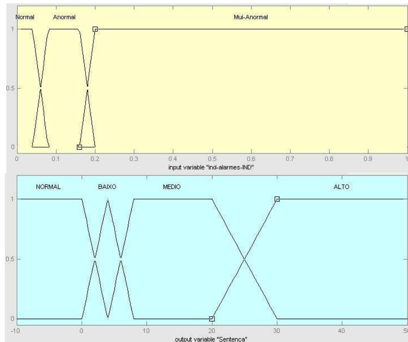
Figura 4.8. Variáveis Nebulosas “ind_alarms_IDI” e “Sentença”.
