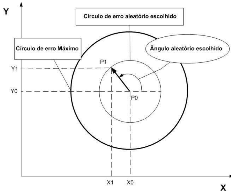
Figura 4.3. Mecanismo de atribuição de erro.
