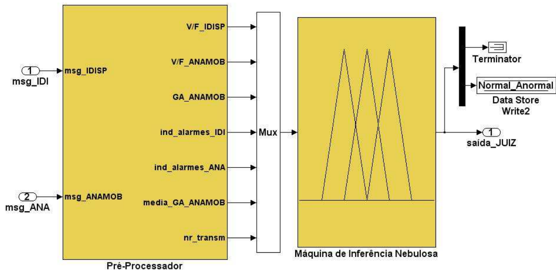
Figura 4.6. O componente "JUIZ".
