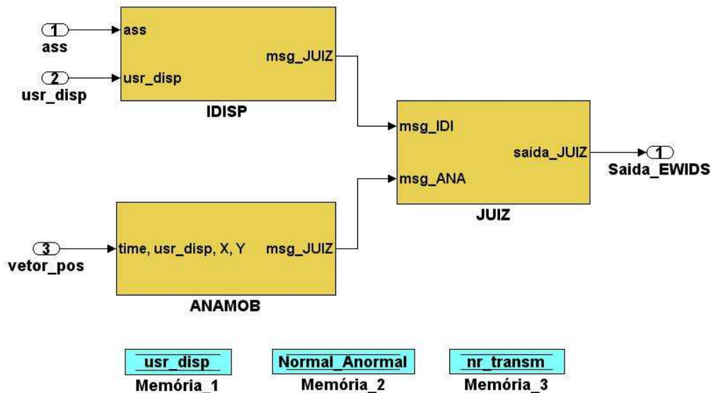
Figura 4.4. Módulos do Protótipo EWIDS.
