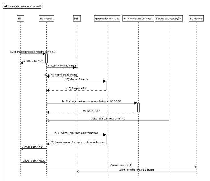
Figura 1. Diagrama de Sequência descrevendo o funcionamento do ARPRAP
